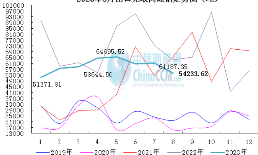
2023年8月出口无取向硅钢走势图（吨）
